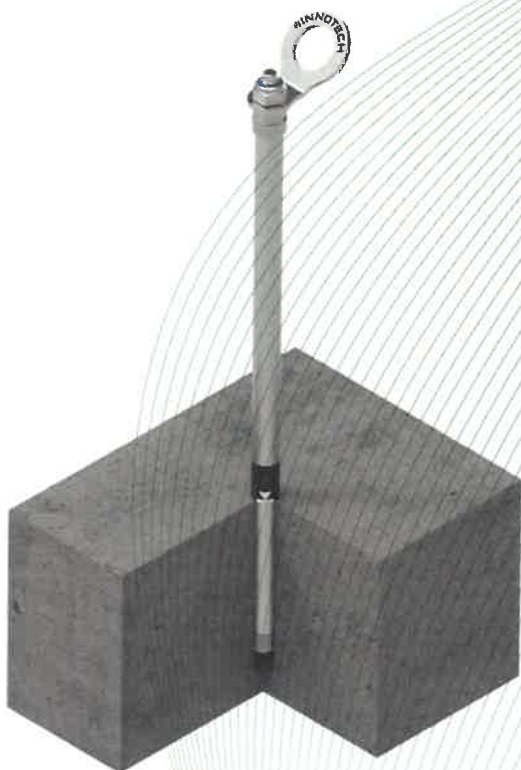
Bild 1: Anschlageinrichtung Typ A, Typ: POINT-12
